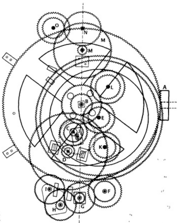
El engranaje de Anticitera (Según el dibujo de B. Pope en Price, Gears, p. 37, fig. 29,
